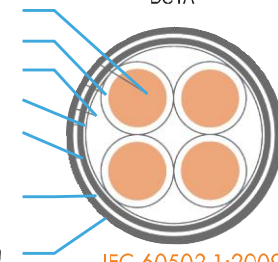
Giáp 2 lớp băng thép Double Galvanized Steel Tape Armoured -DSTA-
