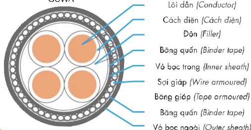
Giáp sợi thép Galvanized Steel Wire Armoured -GSAW-
