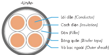
Không giáp Unarmoured -UnAr-
